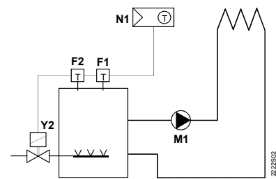
Regulator de temperatură cameră cu comandă directă a unui boiler cu gaz plasat pe pardoseală
